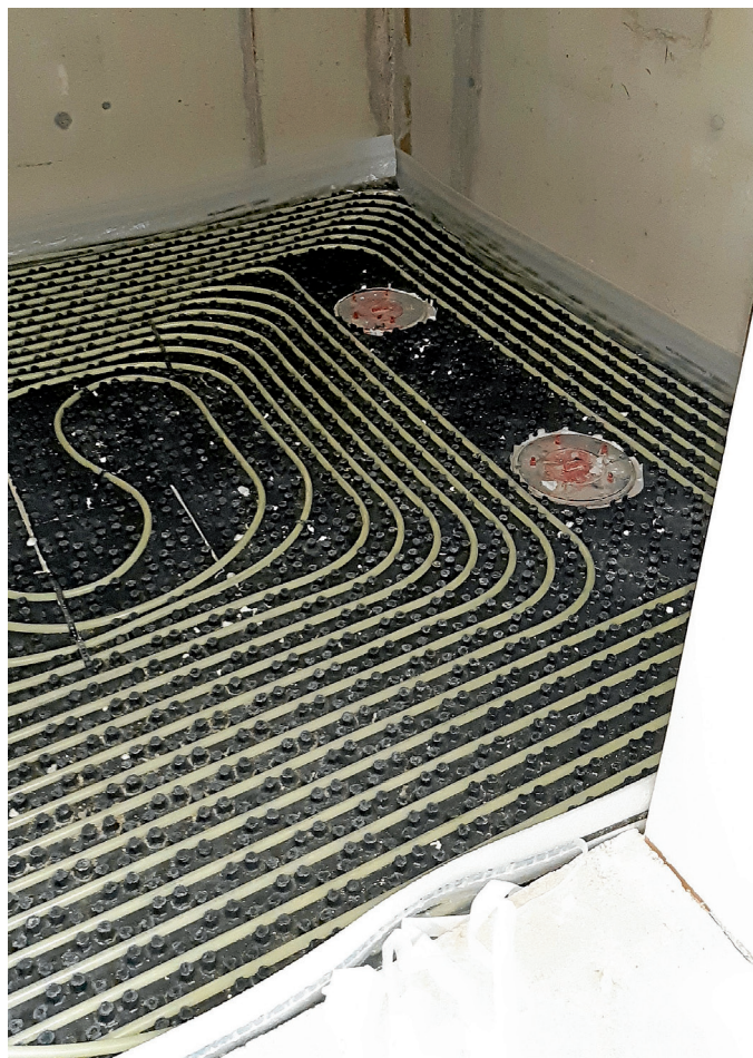
Verlegung der Fußbodenheizung Foto: Neuhäuser Architekten
