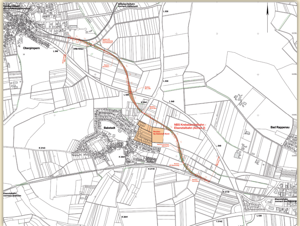
Abbildung: Neubau Verbindungsstrecke Obergimpfern – Bad Rappenau (Plan: VWI Verkehrswissenschaftliches Institut Stuttgart GmbH)
