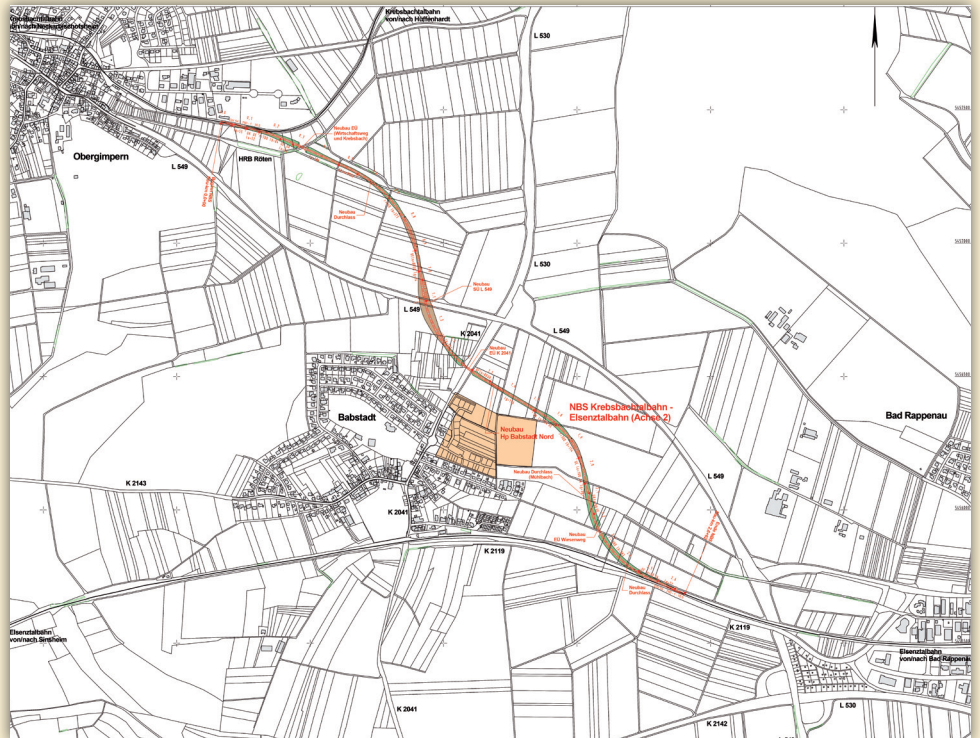
Abbildung: Neubau Verbindungsstrecke Obergimperm – Bad Rappenau (Plan: VWI Verkehrswissenschaftliches Institut Stuttgart GmbH)
